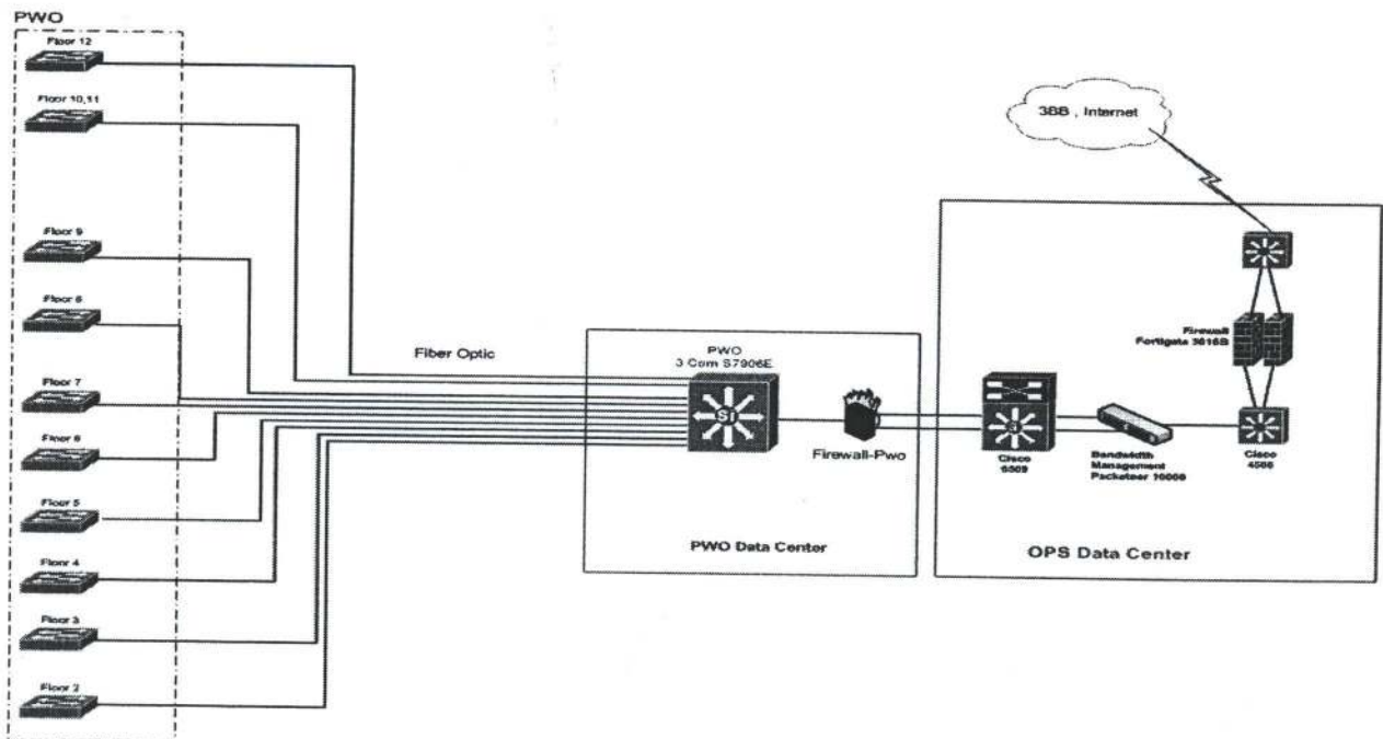
PWO Network Diagram องค์การคลังสินค้า
